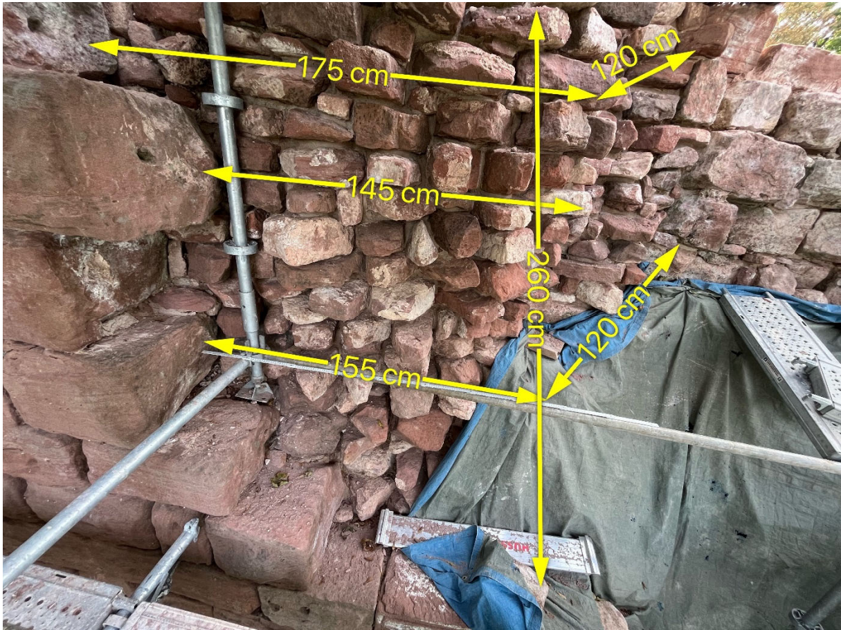
Mur N3 - Colonne de maçonnerie de blocage – reprise en sous-œuvre sous le blocage suspendu conservé
