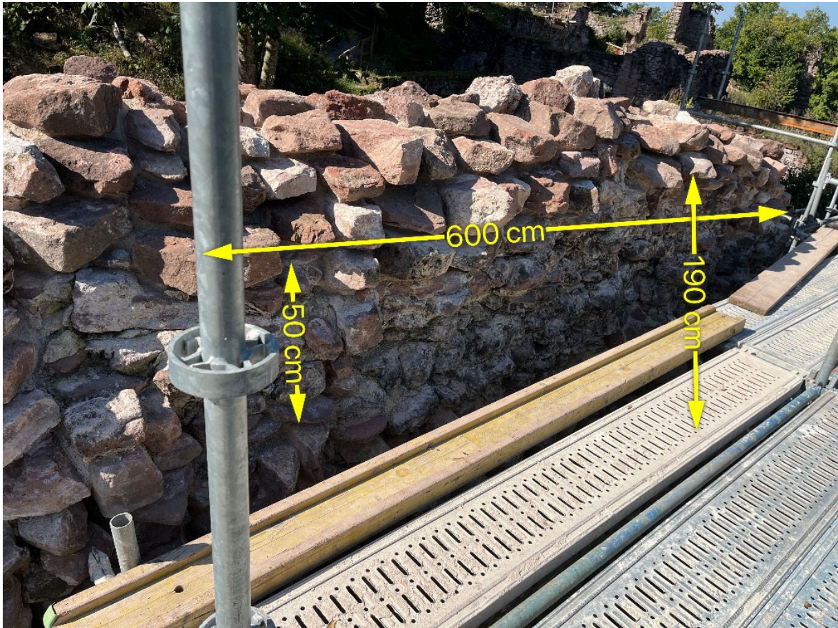
Mur N côté extérieur – Partie de blocage conservée, rejointoyée
