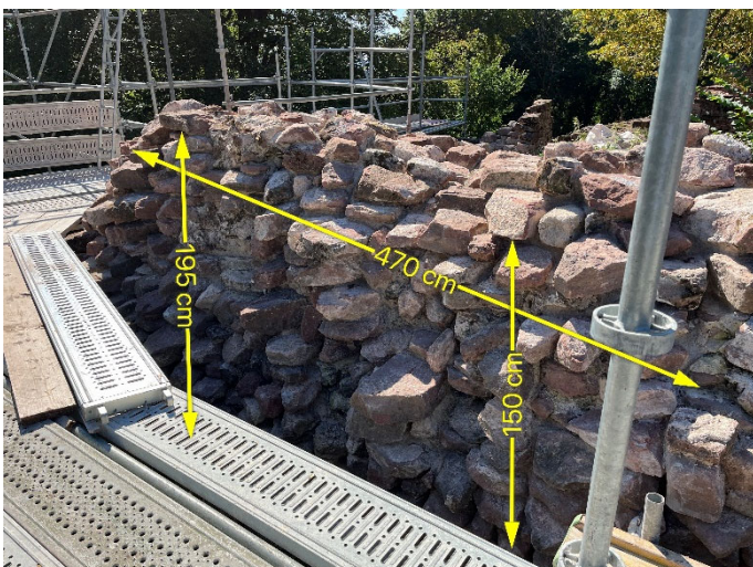
Mur N extérieur – à gauche, arrachement sur toute la hauteur – à droite, arrachement neuf en partie basse...
