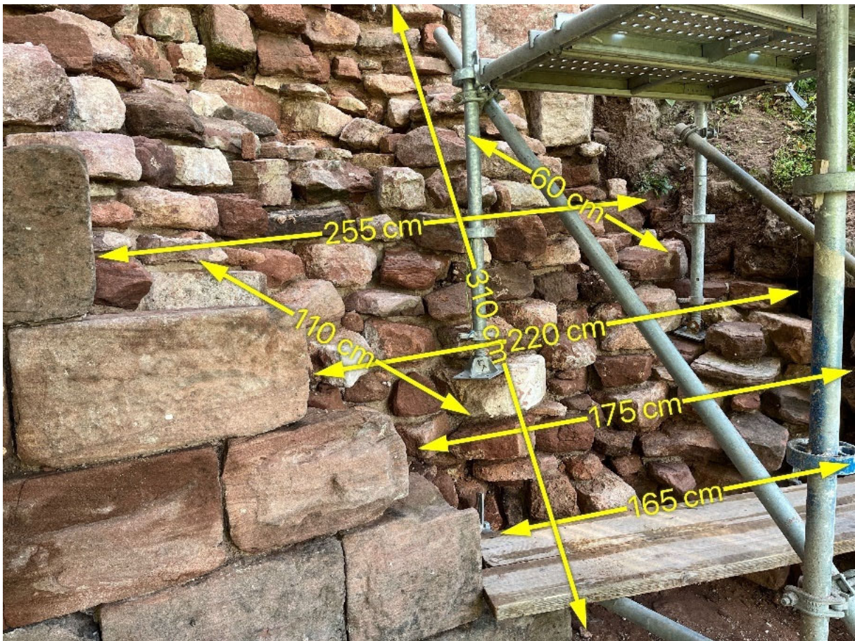
Mur N3 - Maçonnerie de blocage à droite du parement, en pied de mur
